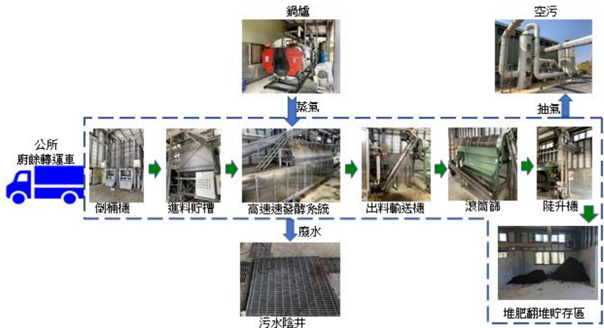
10 噸/日廚餘高速發酵系統處理流程圖
