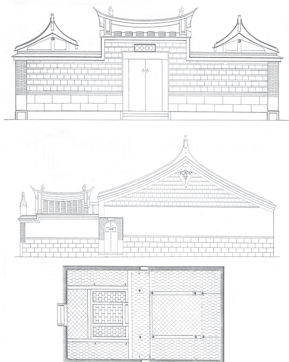
圖 5-3-1-1 一落宗祠之正面、側面、平面
