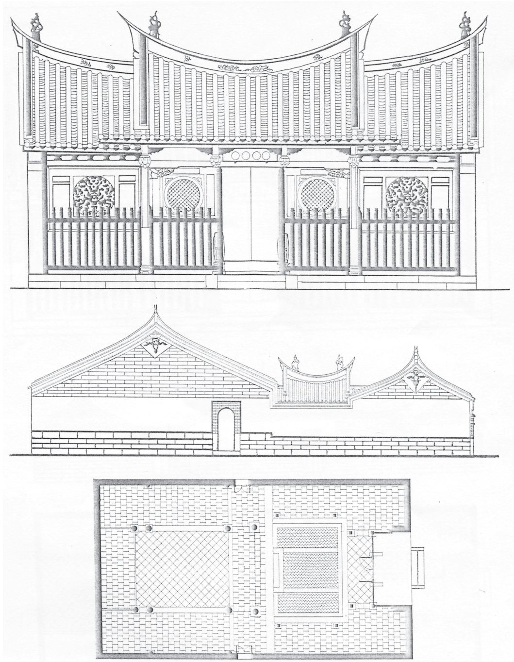
圖 5-3-1-2 二落宗祠之正面、側面、平面
