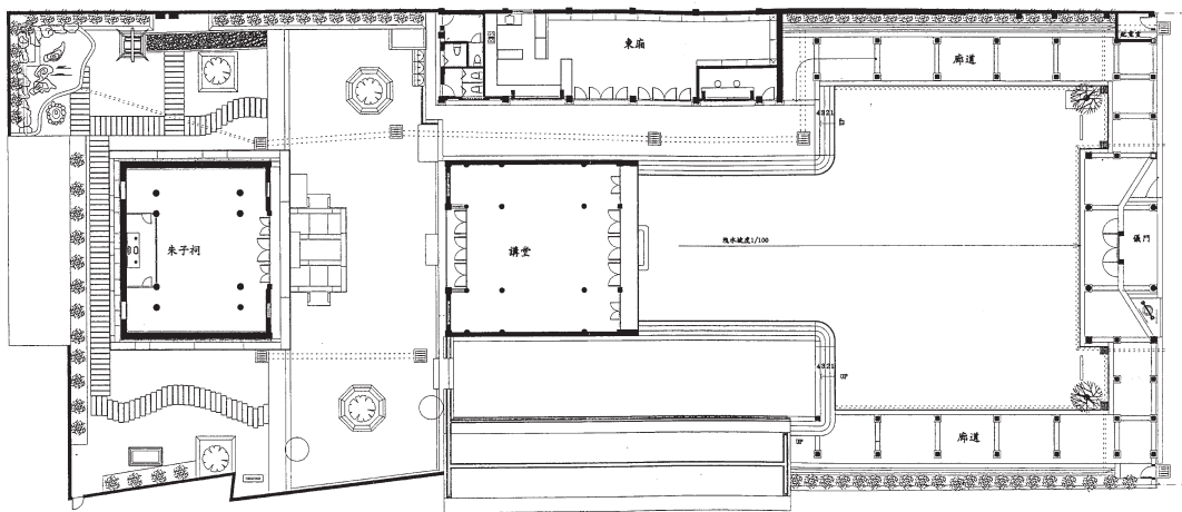
圖 2-3-2-2 浯江書院與朱子祠平面圖
