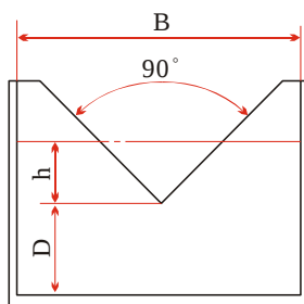
圖 10 直角三角堰
