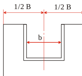
圖 4 四角堰之切口
