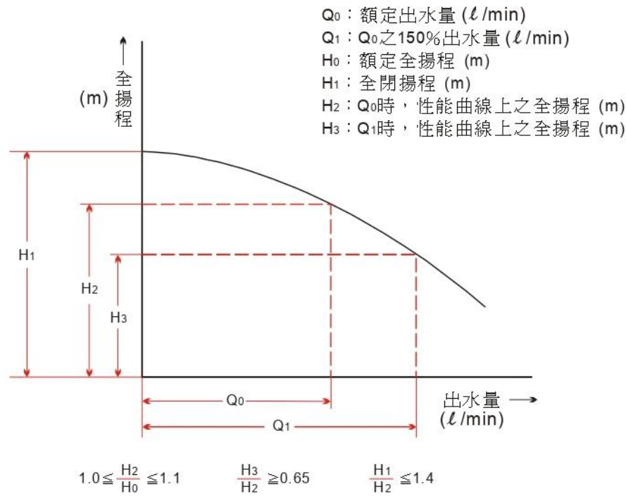
附圖1 性能曲線圖
