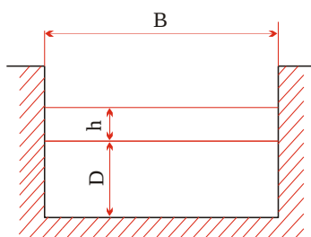
圖 12 全幅堰
