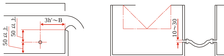
圖 8 堰水頭之測定裝置 (單位：mm)
