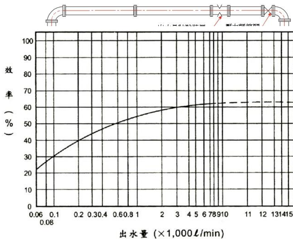
附圖3 幫浦效率曲線
