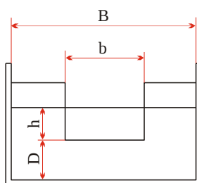
圖 11 四角堰
