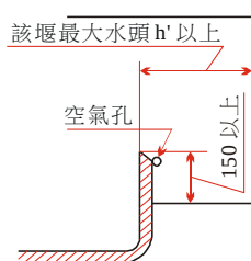
圖 7 全幅堰之水路（單位：mm）
