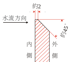
圖 1 堰板之截面圖 (單位：mm)
