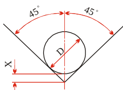
圖 9 三角堰水頭零點之測定
