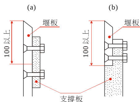
圖 2 堰板之內面圖 (單位：mm)
