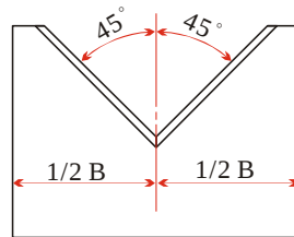
圖 3 直角三角堰之切口
