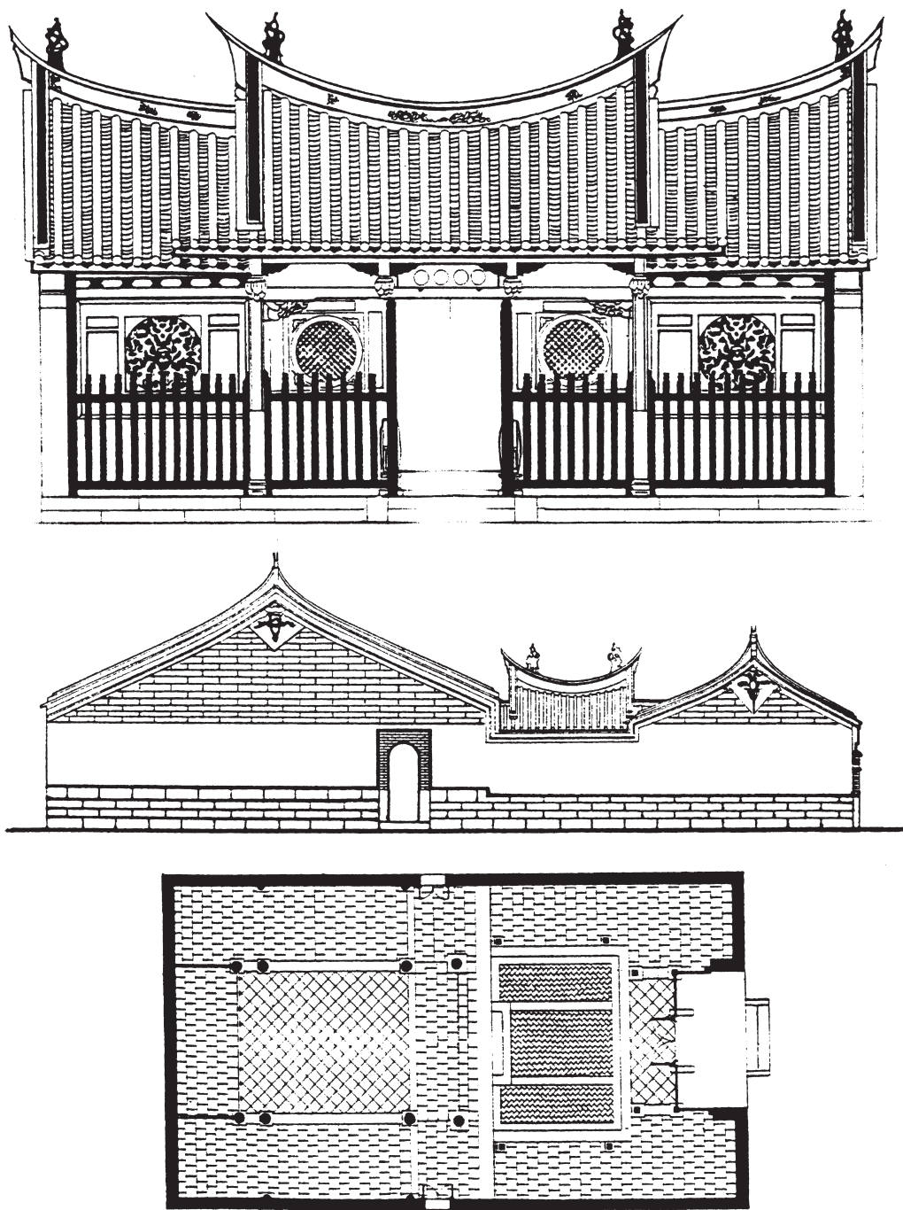
圖二 宗祠二落之正面、側面、平面
