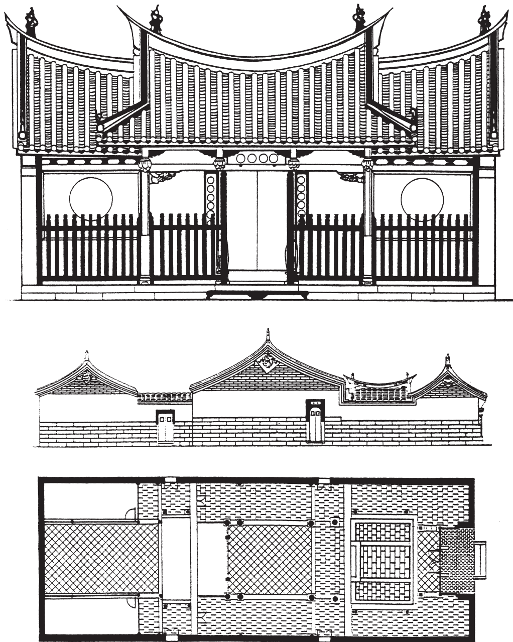
圖三 宗祠三落之正面、側面、平面
