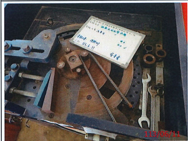
說明：#5鋼筋抗彎試驗中
