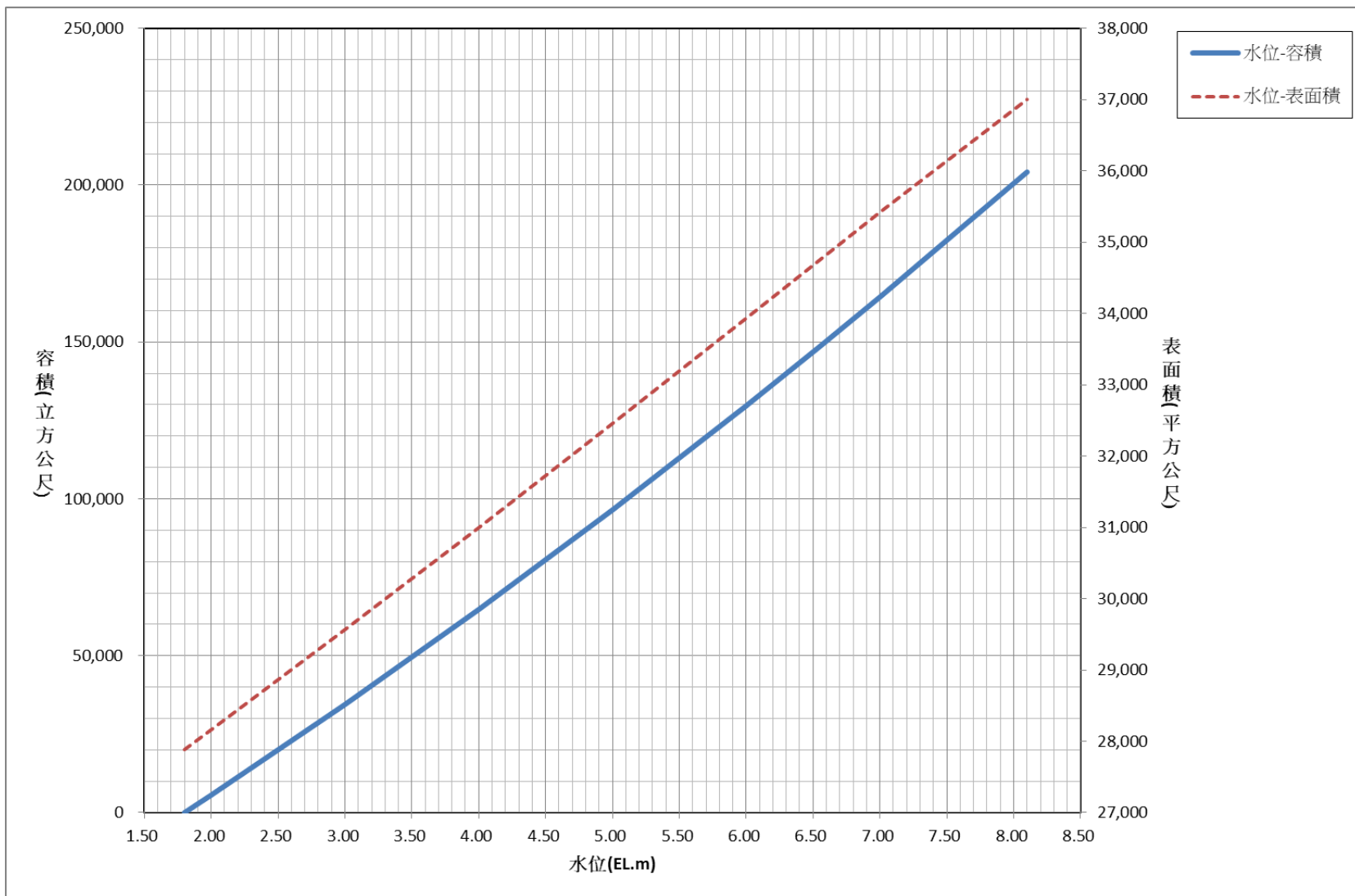
田浦受水池 水位、容積、表面積曲線圖
