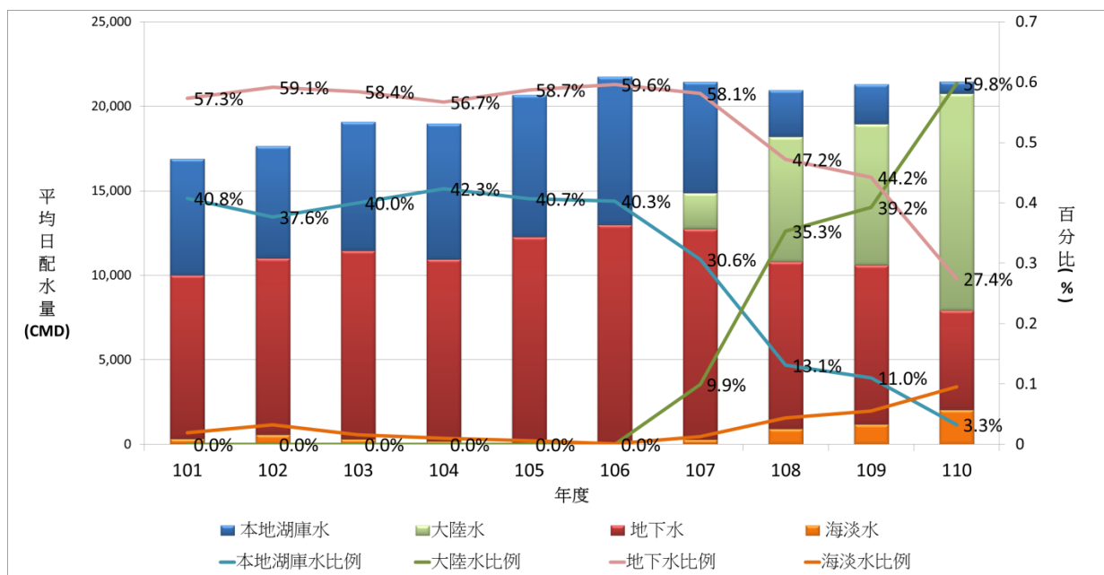
圖 5-1：歷年各類清水出水量分析圖
