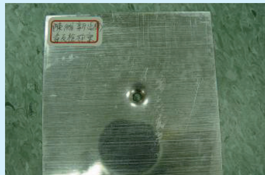
▲貫穿監測鋁板超過單位面積動能16焦耳/平方公分以上
