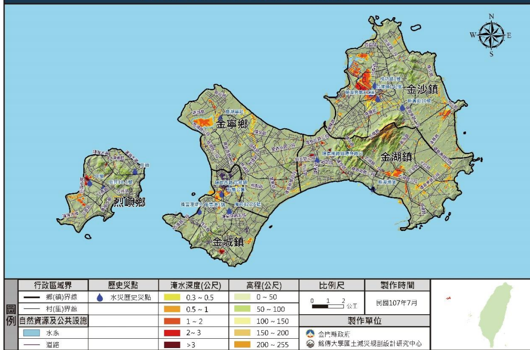
金門縣24小時累積雨量150毫米淹水潛勢圖
