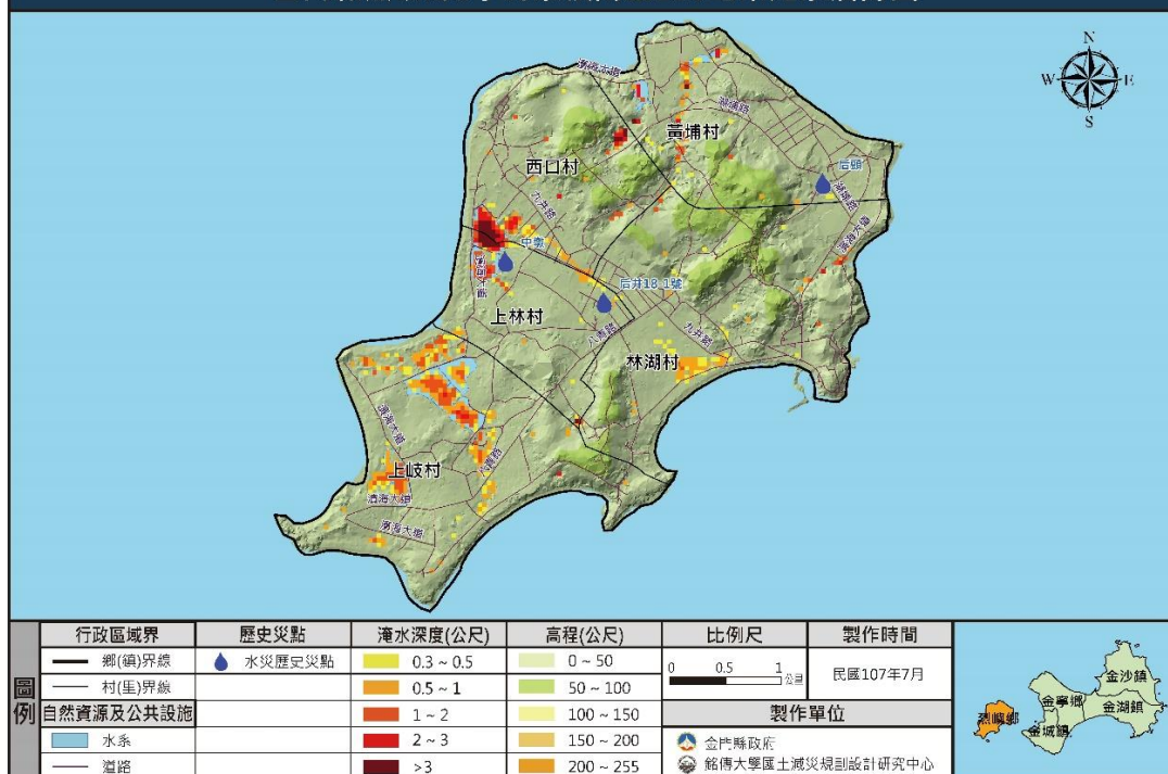
金門縣烈嶼鄉3小時累積雨量130毫米淹水潛勢圖
