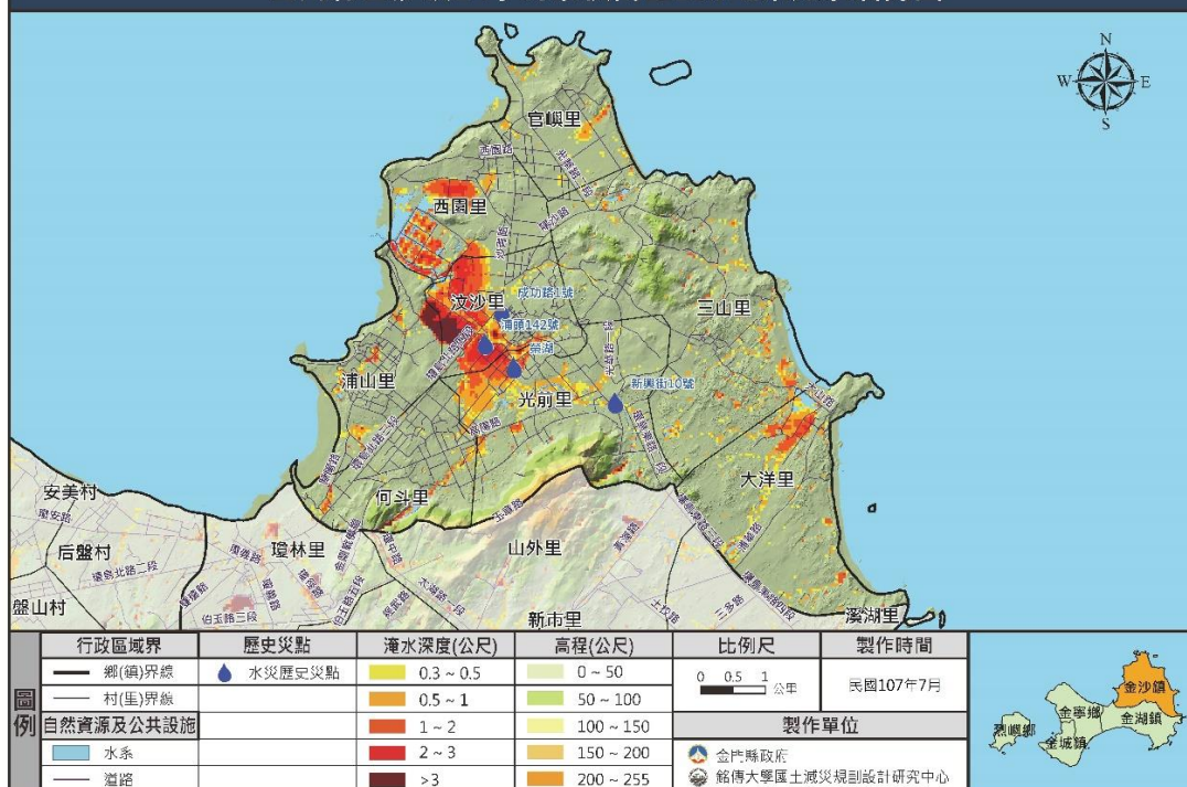
金門縣金沙鎮24小時累積雨量250毫米淹水潛勢圖
