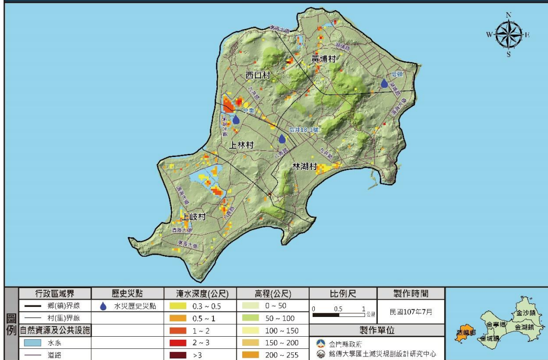
金門縣烈嶼鄉3小時累積雨量60毫米淹水潛勢圖
