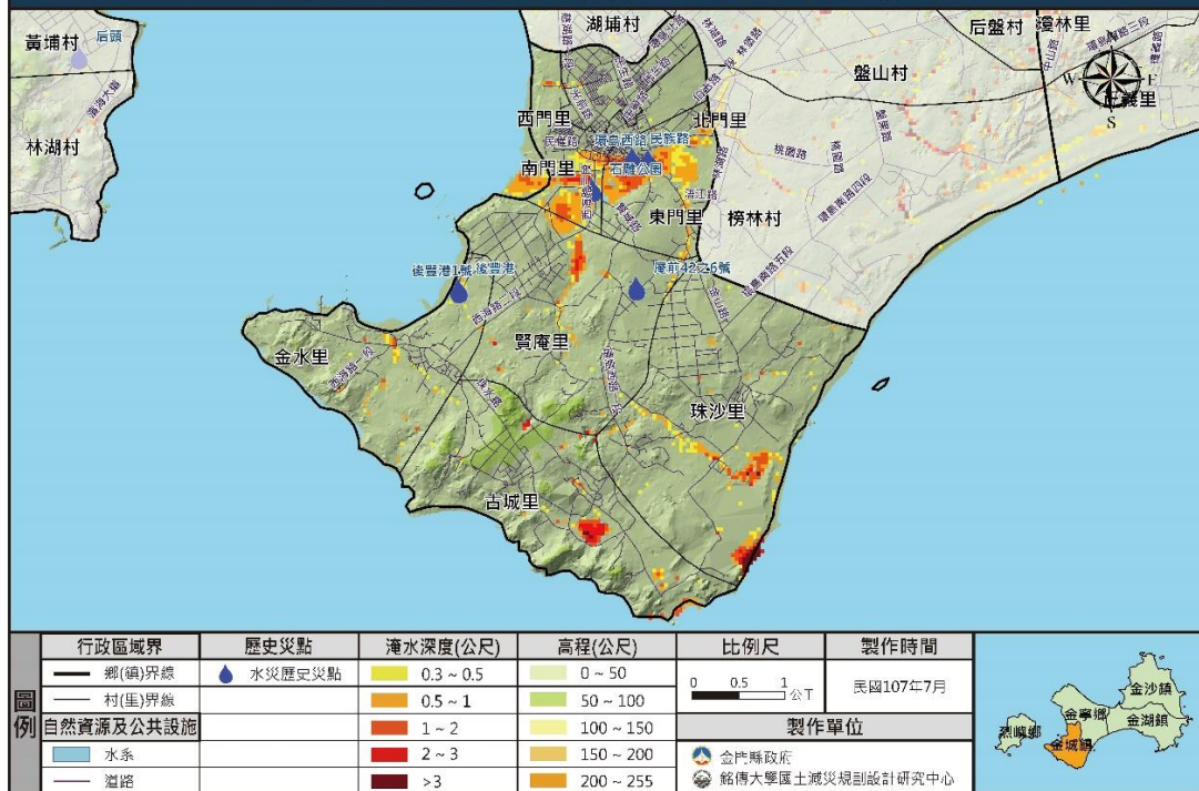
金門縣金城鎮3小時累積雨量120毫米淹水潛勢圖
