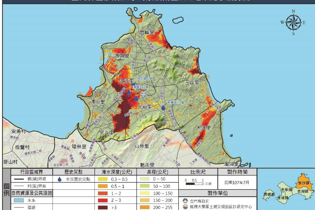
金門縣金沙鎮24小時累積雨量350毫米淹水潛勢圖
