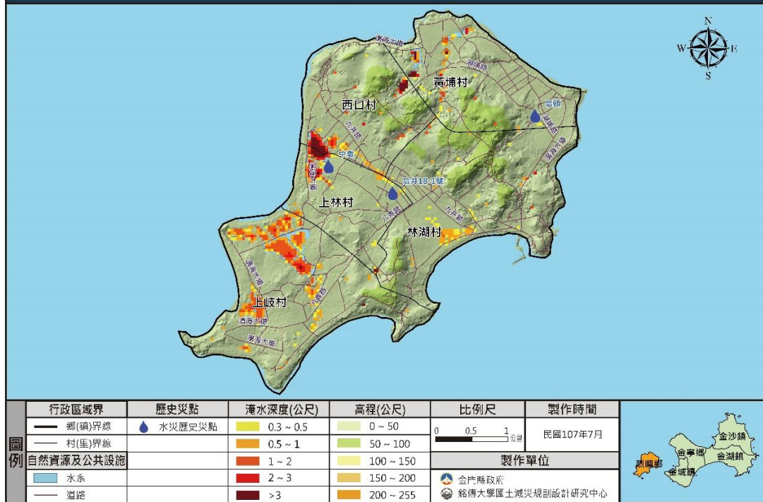
金門縣烈嶼鄉24小時累積雨量250毫米淹水潛勢圖
