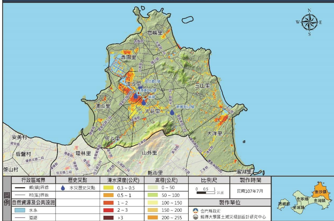
金門縣金沙鎮3小時累積雨量120毫米淹水潛勢圖
