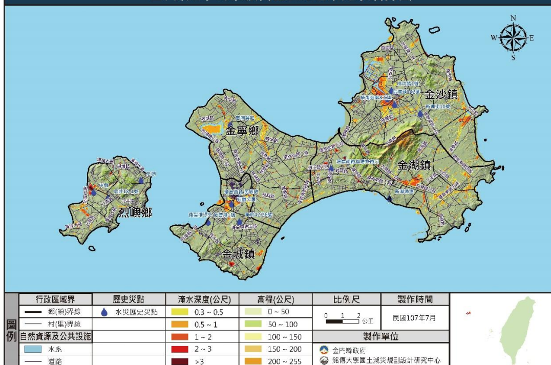
金門縣3小時累積雨量130毫米淹水潛勢圖
