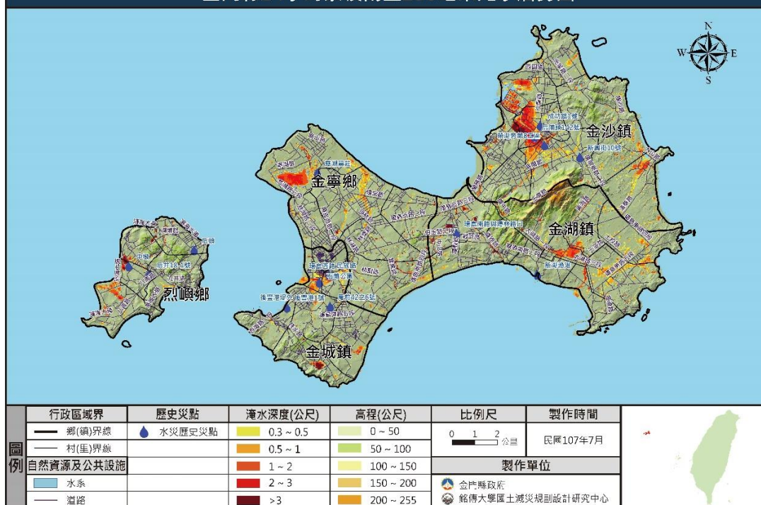
金門縣24小時累積雨量250毫米淹水潛勢圖
