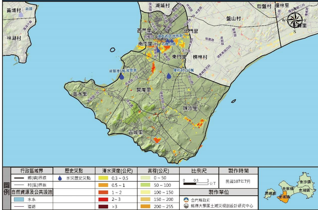
金門縣金城鎮3小時累積雨量60毫米淹水潛勢圖
