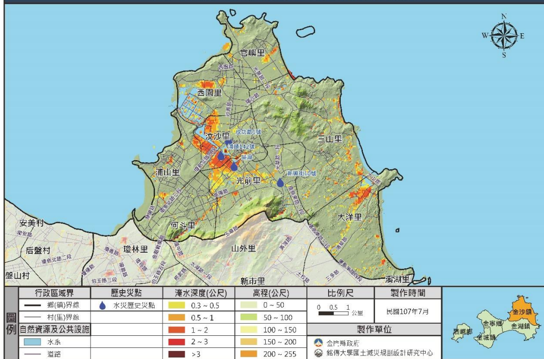
金門縣金沙鎮3小時累積雨量130毫米淹水潛勢圖
